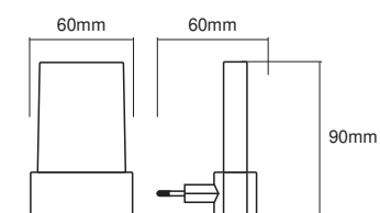
Produkt Line Drawing LUNETTA RGB
