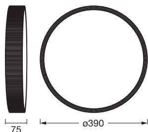
ORBIS MATTEO 390 24W 830CLICKD
