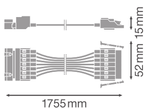
TRUSYS UNIV 1500 7P WIRE
