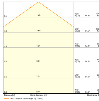
BATTEN CBO 1200 V 36W MS 865 WT
