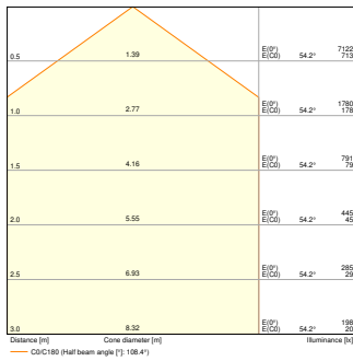
BATTEN CBO 1200 V 36W MS 840 WT
