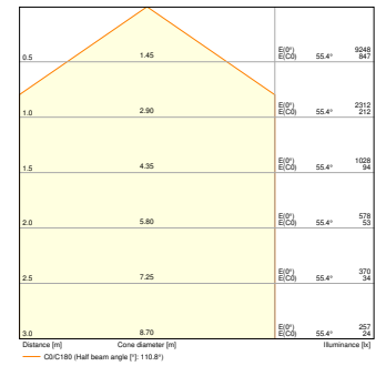
BATTEN CBO 1500 V 48W MS 840 WT
